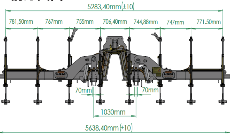
前方図面
