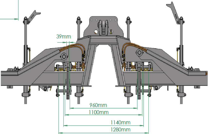
後方図面
