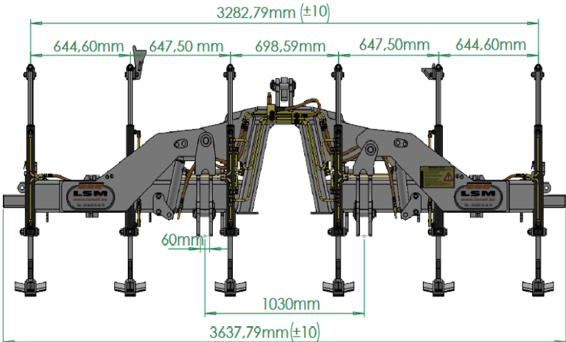
前方図面
