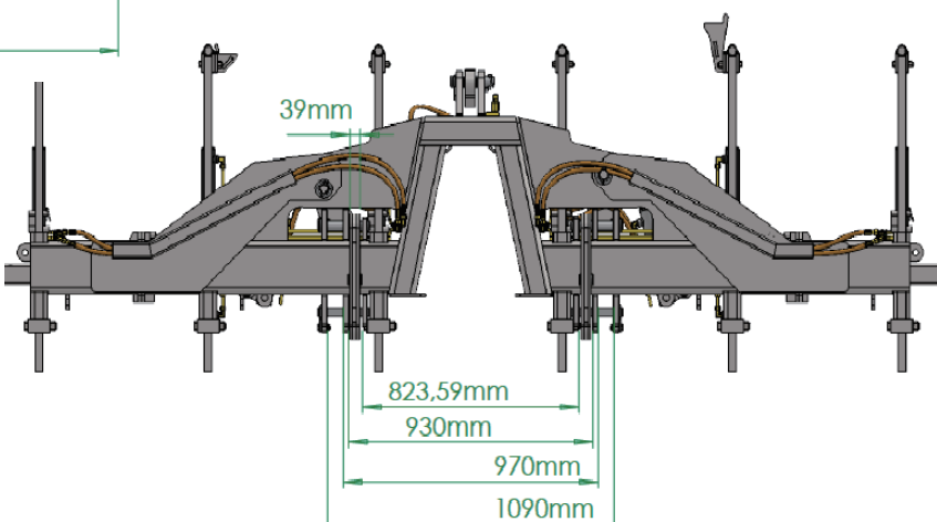
後方図面
