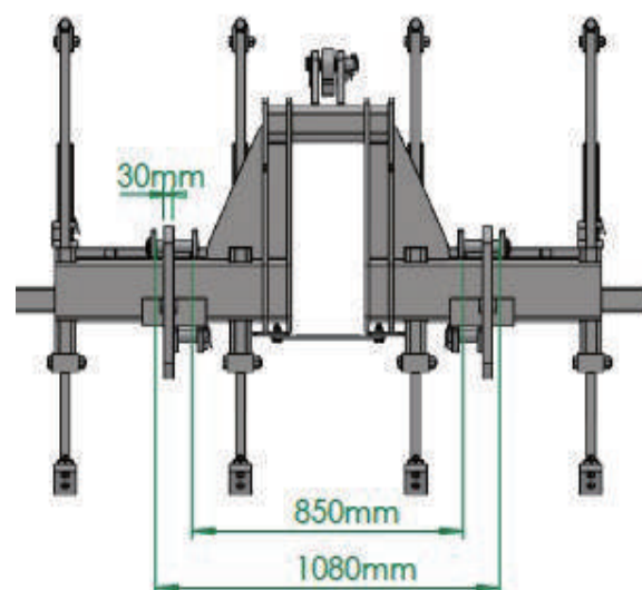
後方図面
