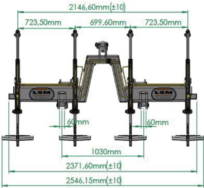
前方図面
