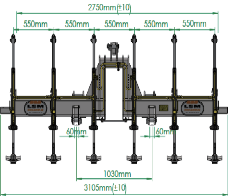
前方図面
