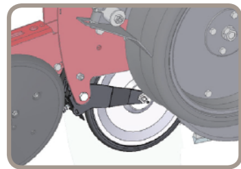
プレスホイール ダブルディスクコルターとV クローリングホイールの間に取付けられ種子 と土を密着して発芽を促進します
