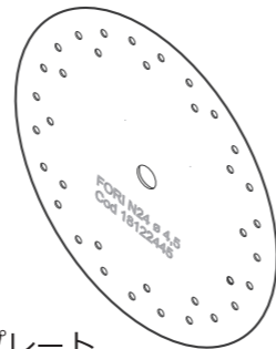
シードプレート 種子の大きさ、株間に合わせて選択してください
